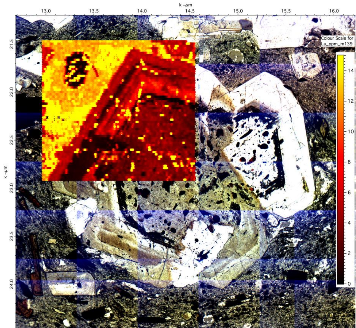
1.1. ábra: A La-koncentráció változása a Kis-Haram plagioklász fenokristályán belül
