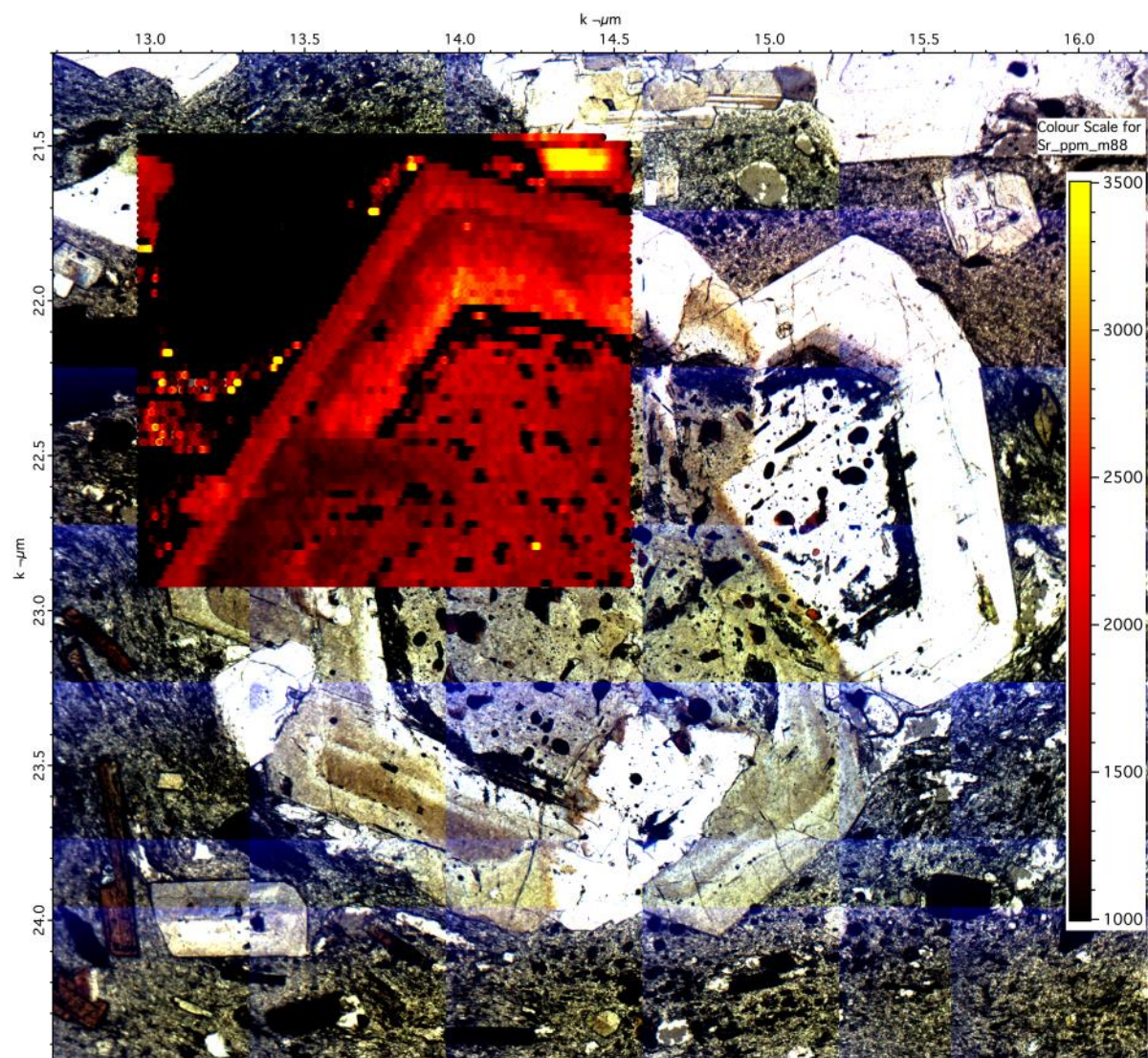
1.2. ábra: A Sr-koncentráció változása a Kis-Haram plagioklász fenokristályán belül
