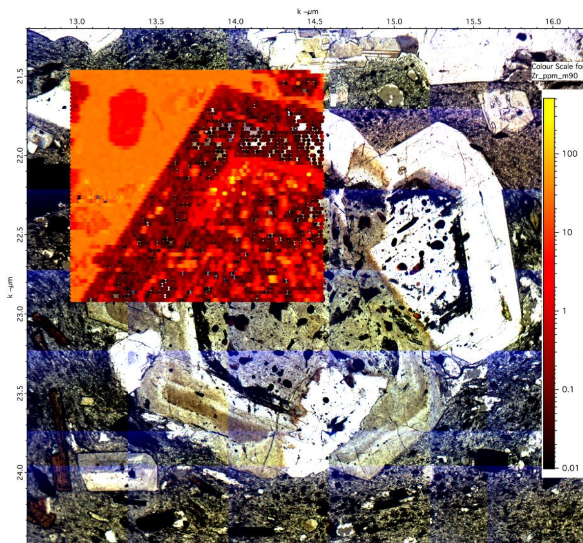
1.3. ábra: A Zr-koncentráció változása a Kis-Haram plagioklász fenokristályán belül
